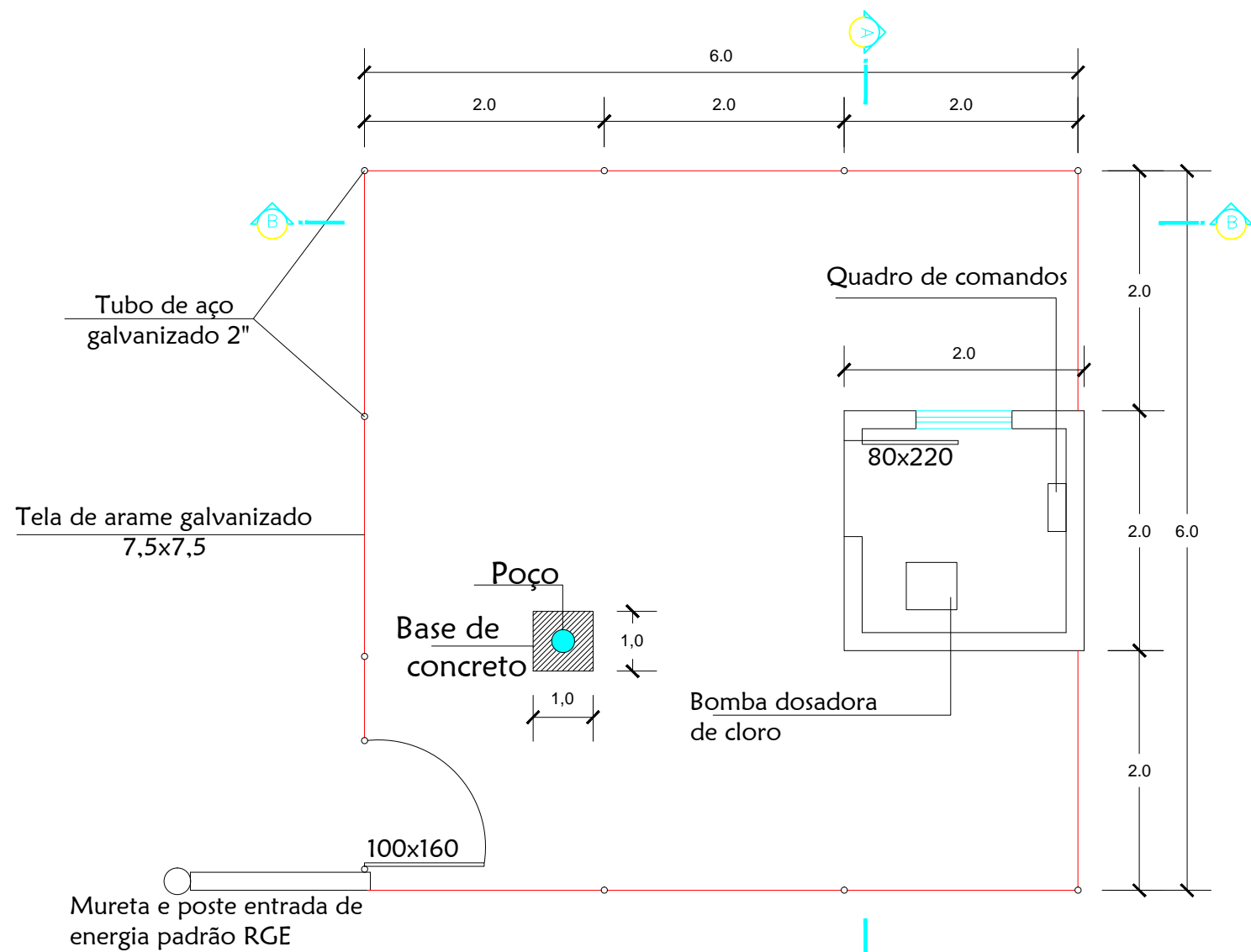
PLANTA BAIXA CERCAMENTO DO POÇO E ABRIGO
