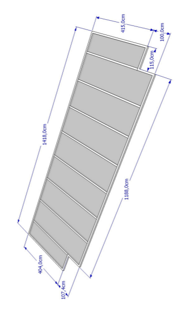
ESTRUTURA METÁLICA COBERTURA PÁTIO COBERTO
