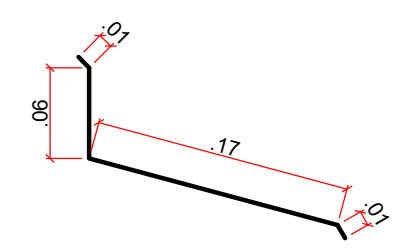
2 DETALHE RUFO Escala 1:5
