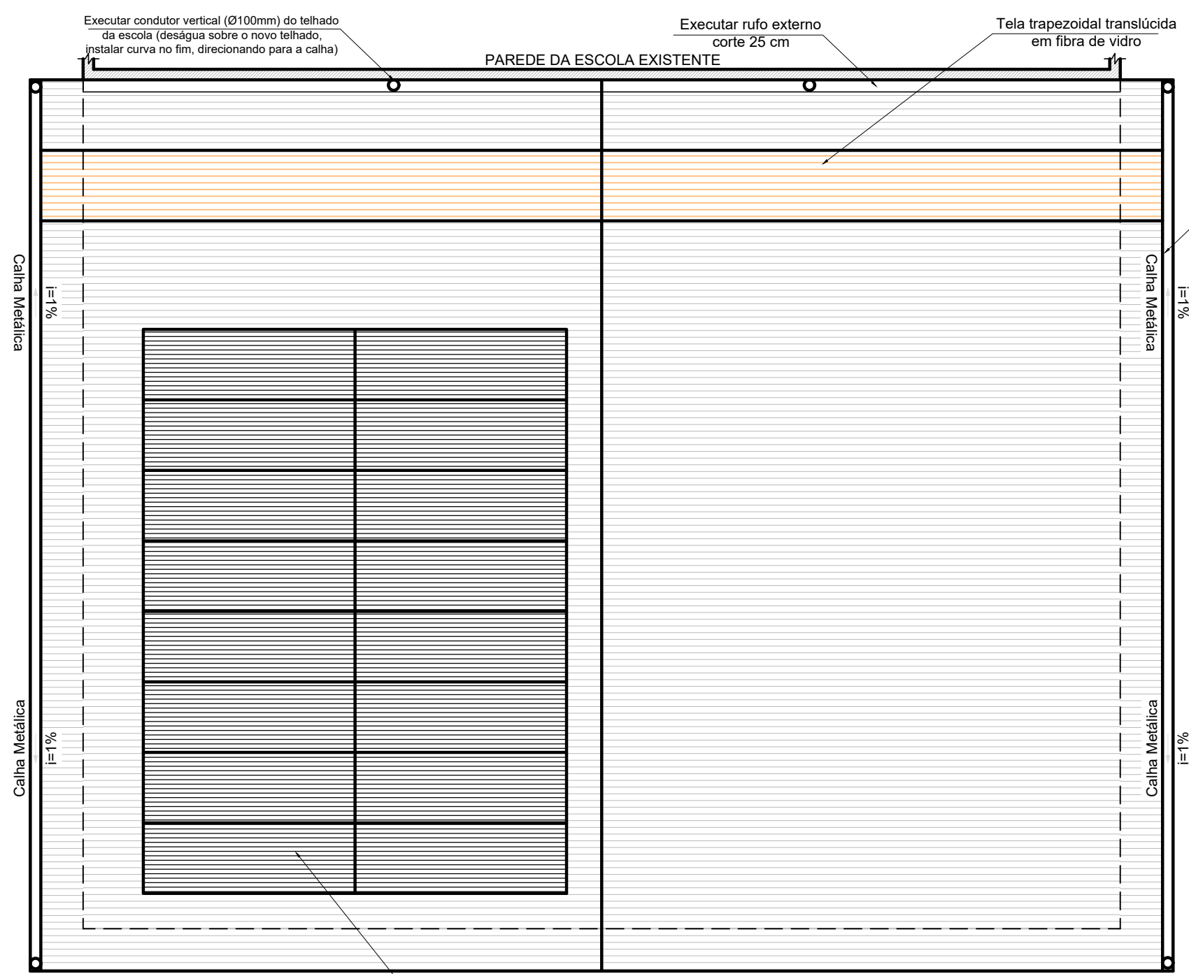
1 COBERTURA Escala 1:75
