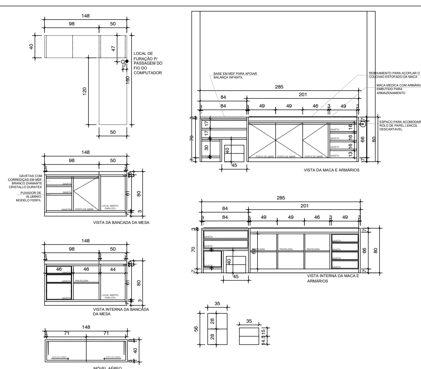
VISTA CONSULTÓRIO 1
