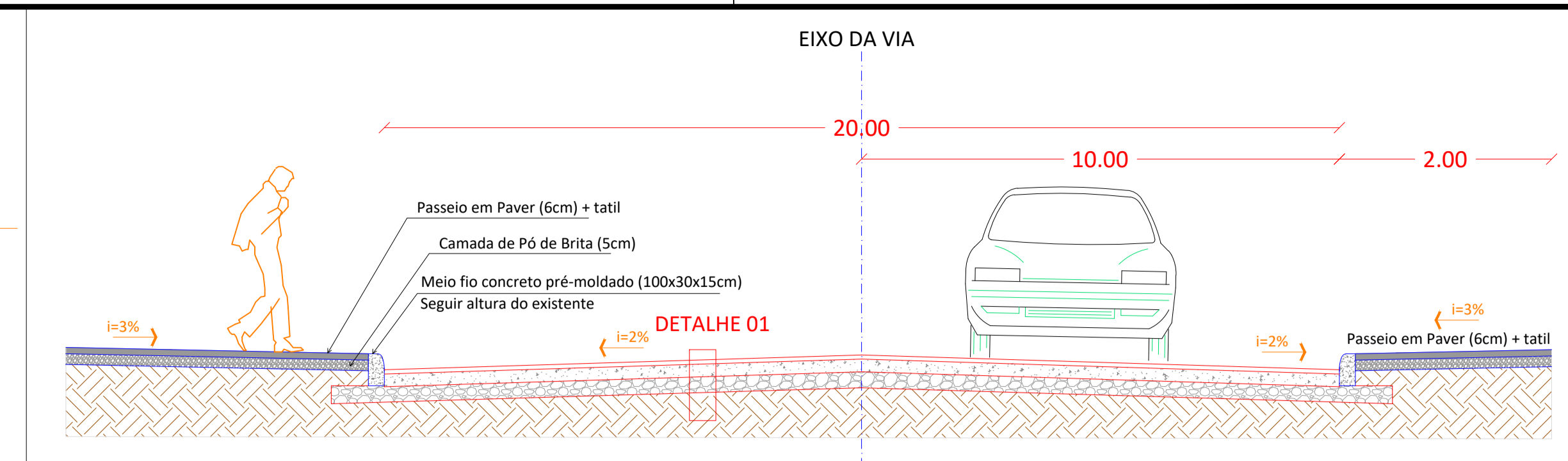
Detalhe esquemático da Rua
