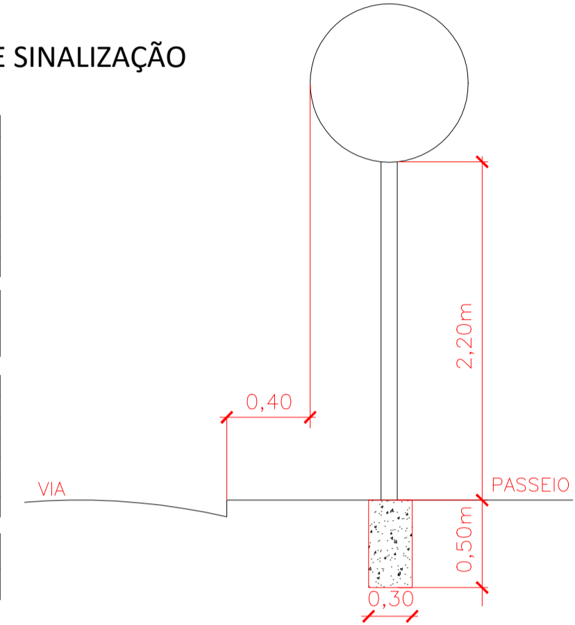
DETALHE 03- LOCAÇÃO DE PLACAS DE SINALIZAÇÃO Sem escala
