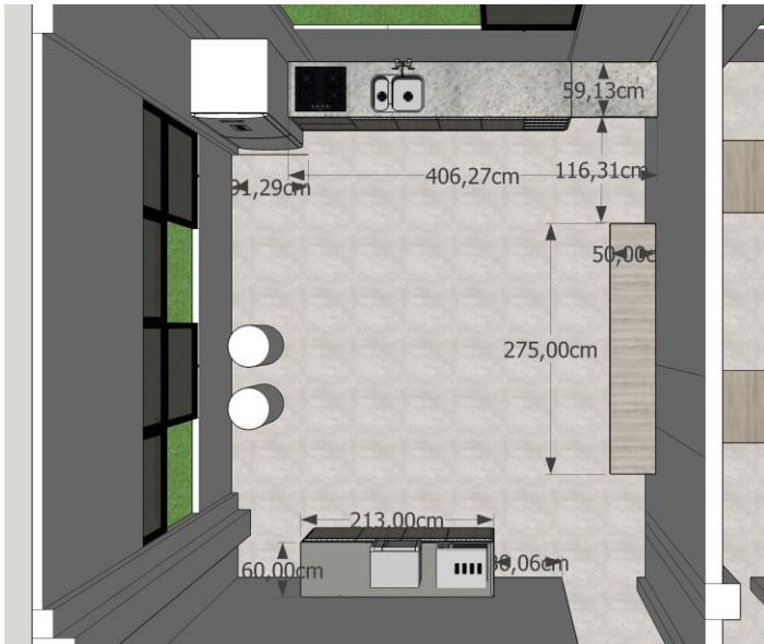
VISTA LOCAÇÃO MÓVEIS COZINHA.
