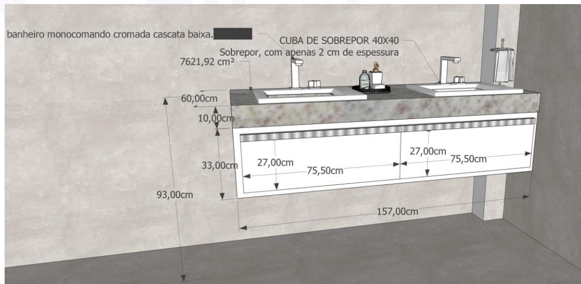
VISTA DO BANHEIRO MASCULINO.
