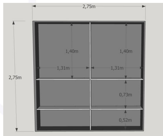
VISTA ARMÁRIO INTERNO SALA TI.
