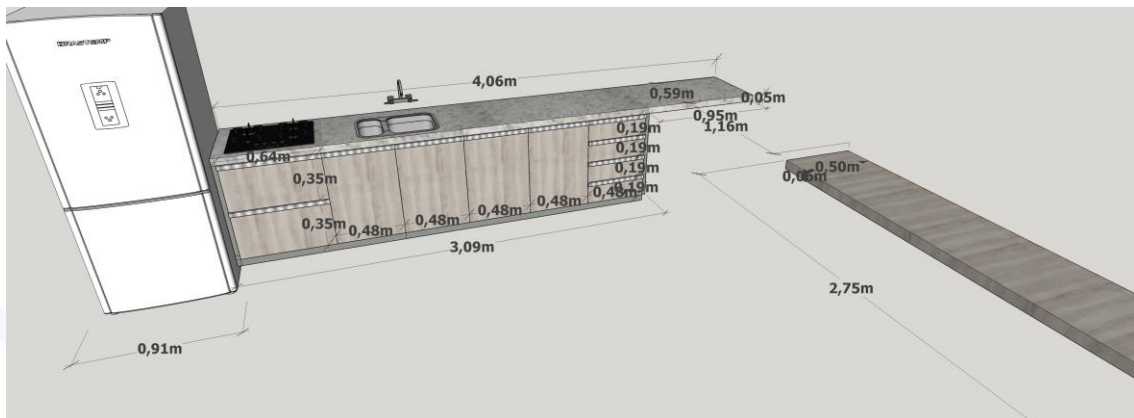
VISTA LOCAÇÃO MÓVEL2 COZINHA.
