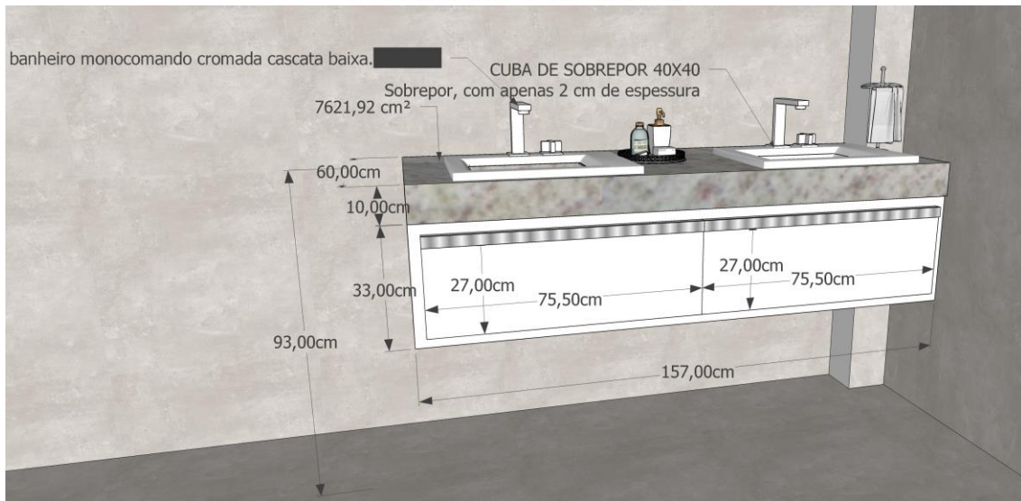
VISTA DO BANHEIRO FEMININO.
